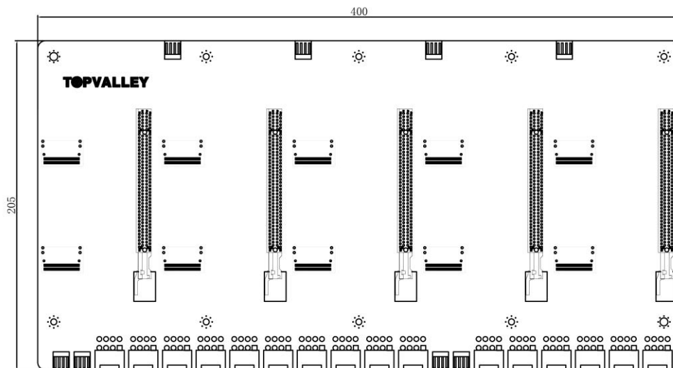
GPU 底板结构图
